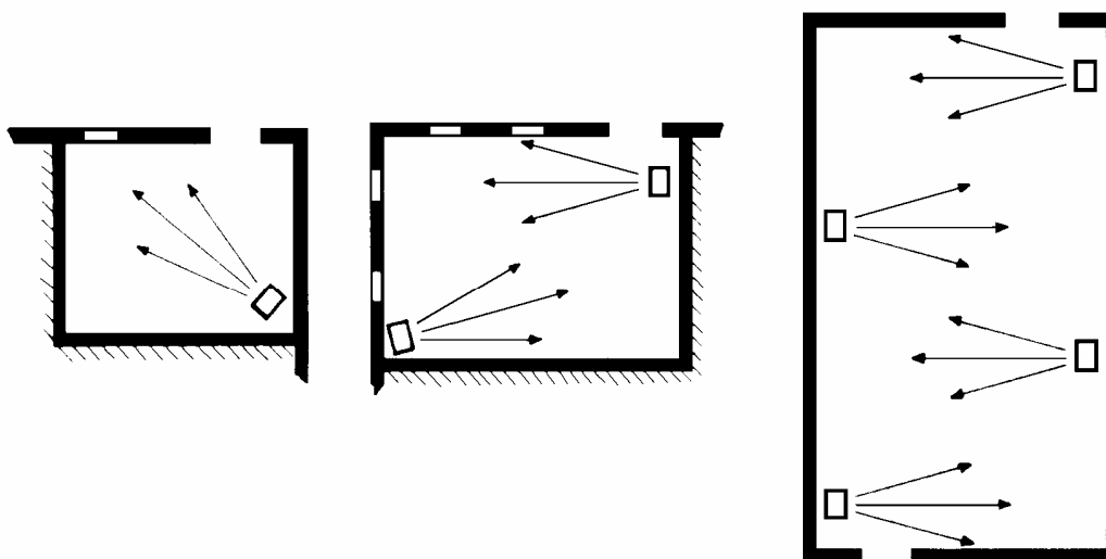
Рисунок 15 – Пример расположения воздухонагревателей
