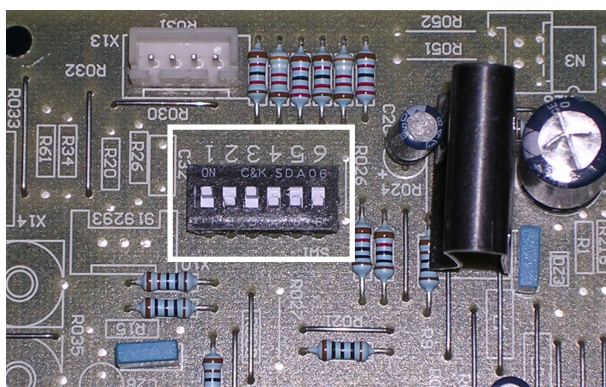
Рисунок 40 – Положение минипереключателя DIP на схеме
