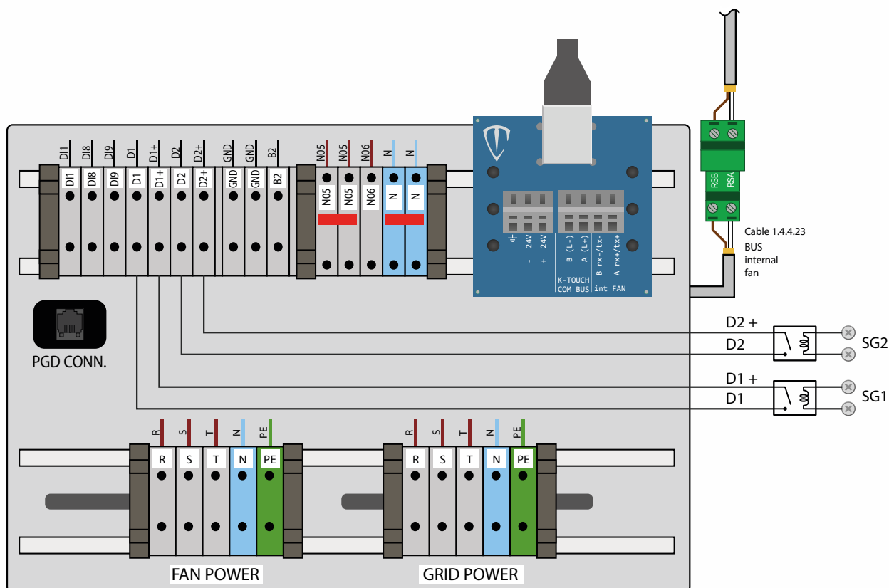
FIG. 19 (SG-Ready protocol)
